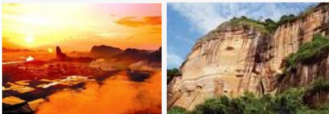
江西龙虎山国家地质公园
